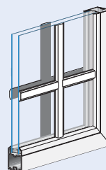
SDL
